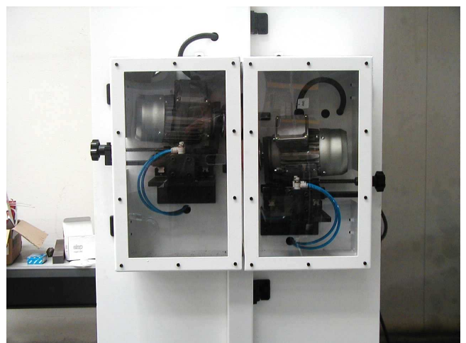
Affilatore motorizzato Motorized grinding unit
